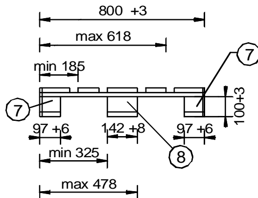
Vue transversale
