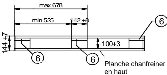
Vue longitudinale
